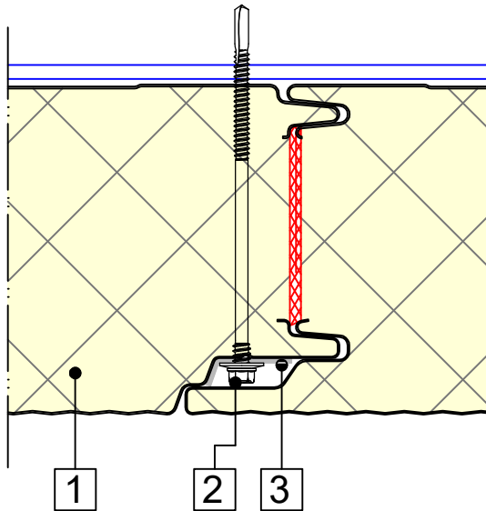
Horizontale doorsnede
