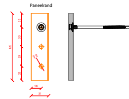
Drukverdeelplaat Alpha-AR Afmeting: 120* 31* 9* 1,5 Artikelnr.: 1008906
