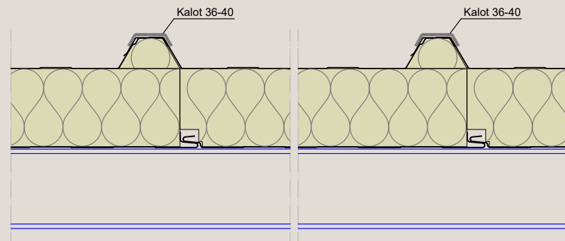
Doorsnede A-A
